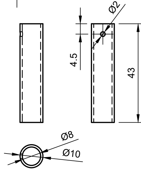
Cylindre laiton
