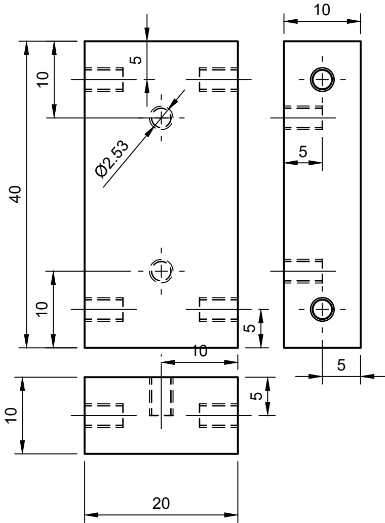
Entretoise alu
