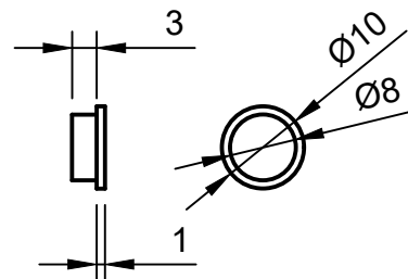
Bouchon
