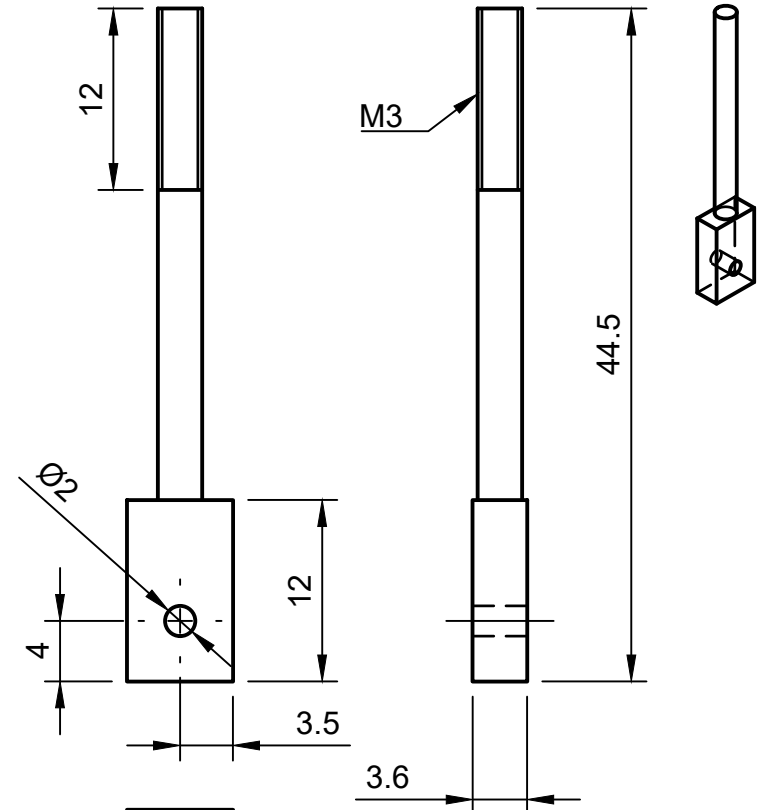
Bielle Ech 2
