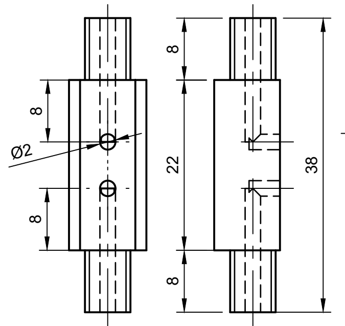
Cylindre laiton
